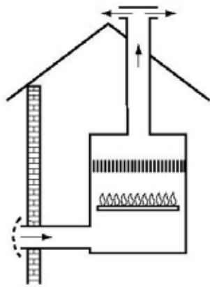
C52 με ανεμιστήρα μετά τον εναλλάκτη θερμότητας
