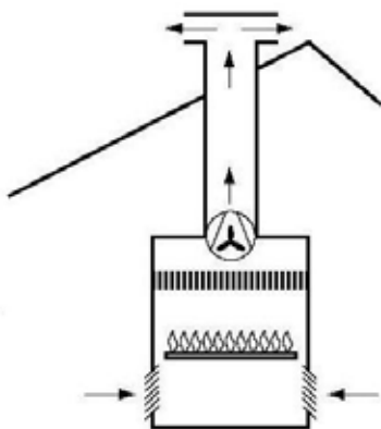
B53 με ανεμιστήρα πριν τον καυστήρα
