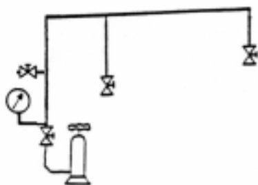
Εικόνα 10.2 Δοκιμή στεγανότητας
