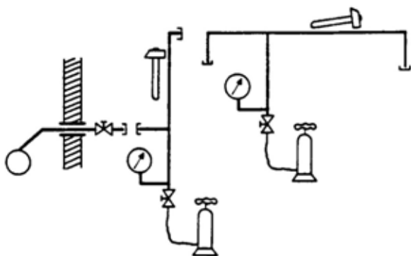
Εικόνα 10.1 Δοκιμή αντοχής
