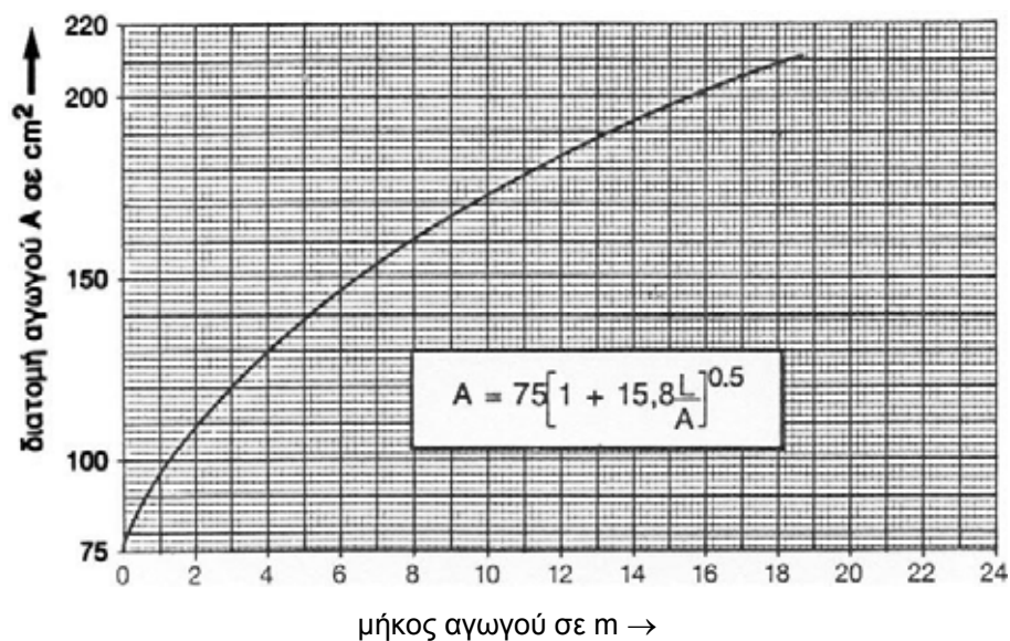
Διάγραμμα 8.2 Ισοδύναμη τετράγωνη διατομή αγωγού για αγωγό ελεύθερης διατομής 75 cm 2 εξαρτώμενη από το μήκος του αγωγού L
