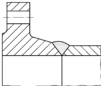
Εικόνα 1.4 Συνιστώμενες κατατομές συγκολλήσεων φλαντζών
