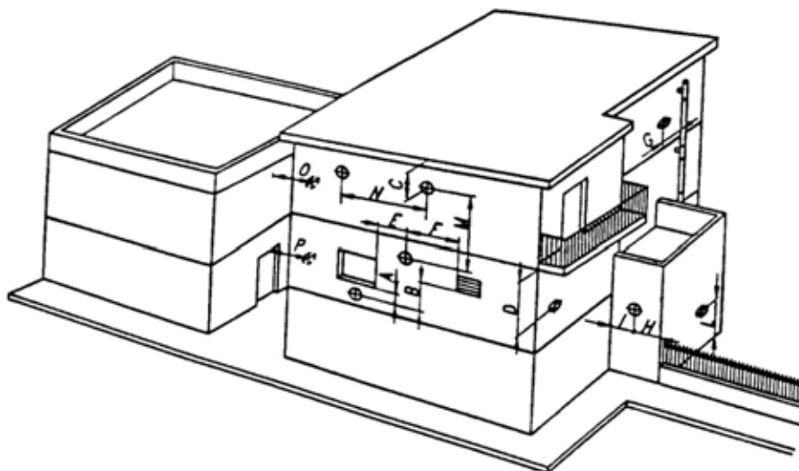
Εικόνα 8.6 Αποστάσεις στομιών συσκευών αερίου
