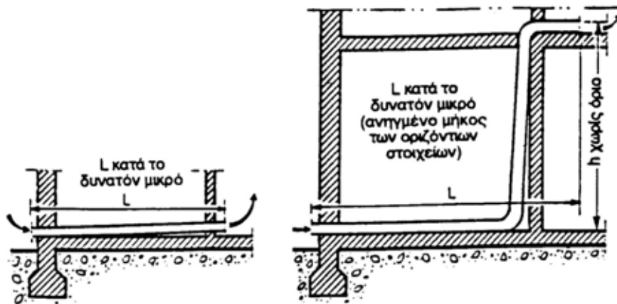
Εικόνα 8.4 Παραδείγματα οδήγησης αγωγών τροφοδοσίας αέρα
