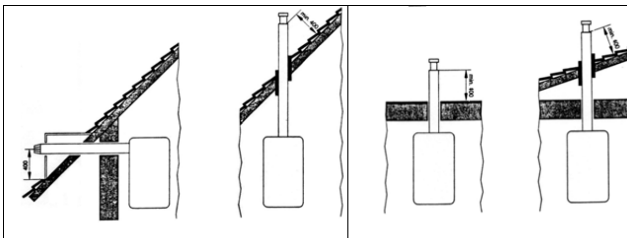
Εικόνα 8.7 Παραδείγματα για την οριζόντια και κατακόρυφη οδήγηση του αγωγού προσαγωγής αέρα και απαγωγής καυσαερίων επάνω από τη στέγη
