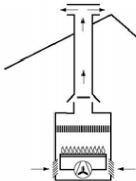
B43 με ανεμιστήρα πριν τον καυστήρα
