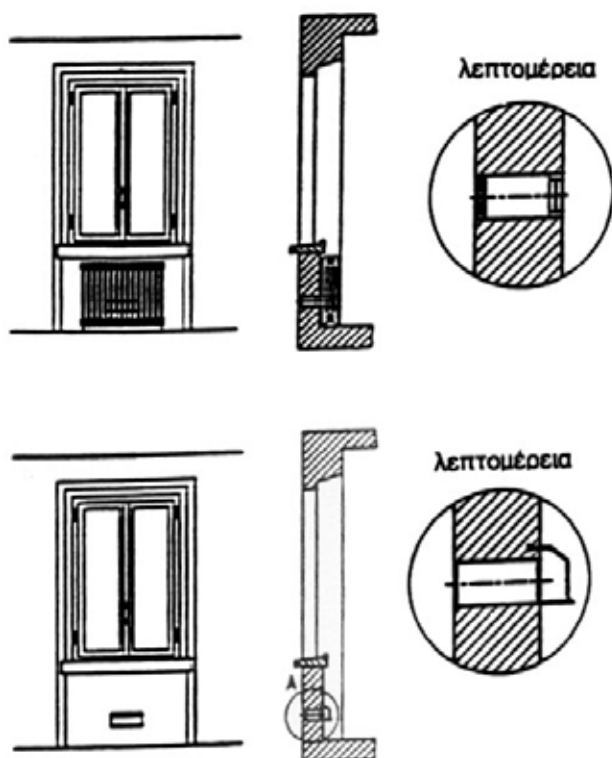
Εικόνα 8.3 Παραδείγματα θέσεων ανοιγμάτων τροφοδοσίας αέρα
