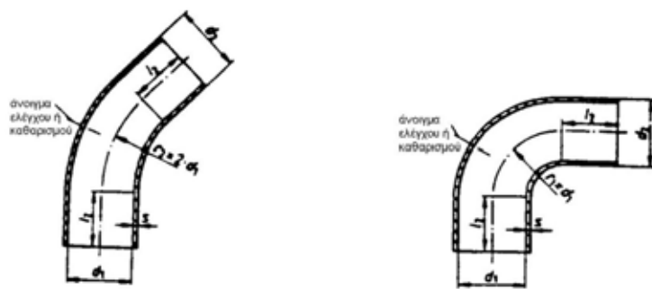
Εικ.9.4 Στοιχεία μορφής καπναγωγών από μέταλλο
