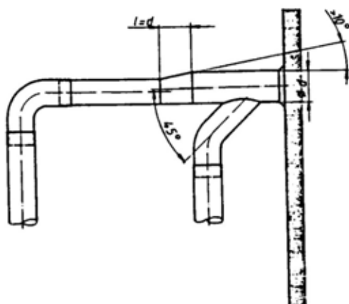
Εικόνα 9.1 Σχεδιασμός κοινού καπναγωγού
