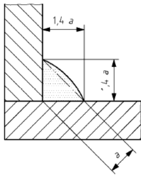
Εικόνα 1.3 Διαστάσεις εξωρραφών
